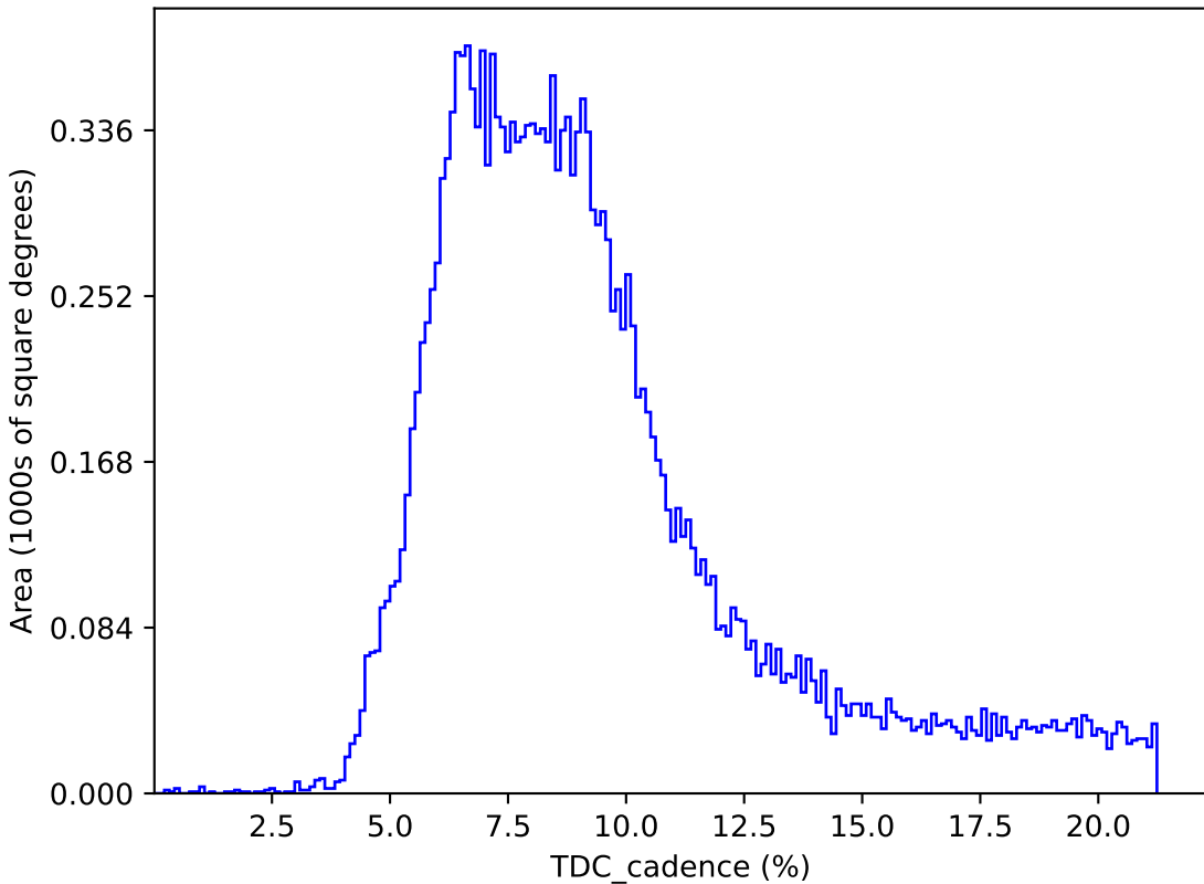
too_10_1v3.4_10yrs : TDC_cadence
