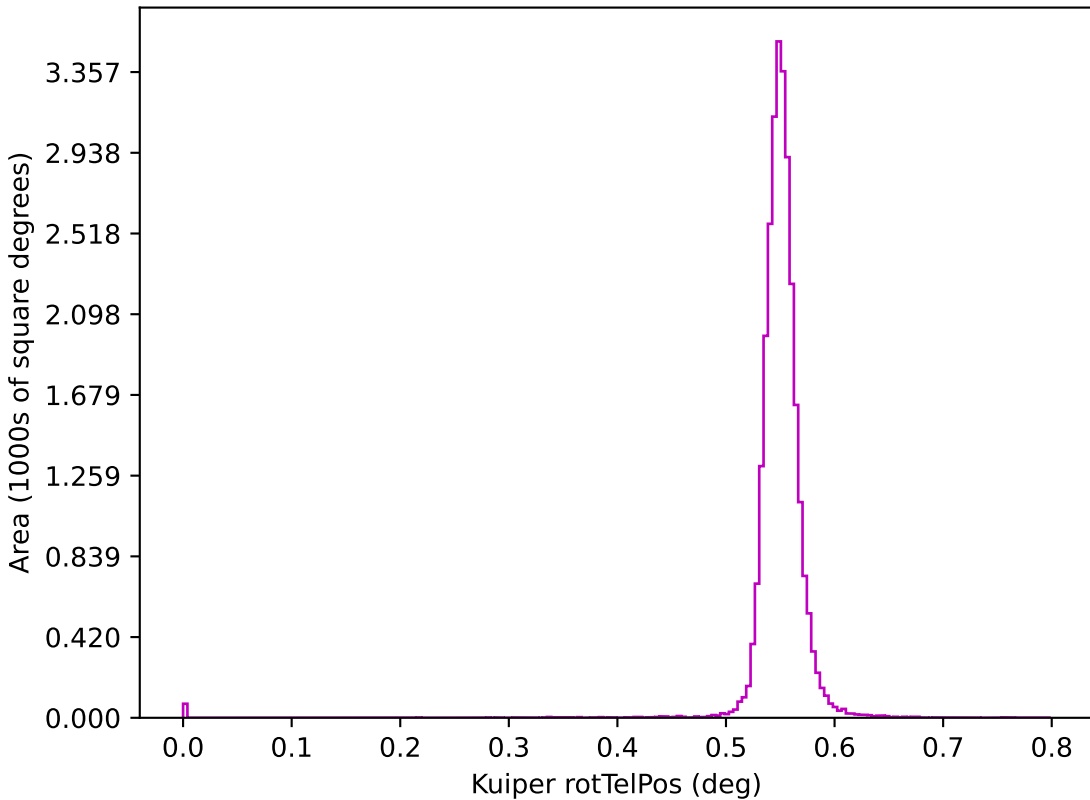
too_10_1v3.4_10yrs z: Kuiper rotTelPos
