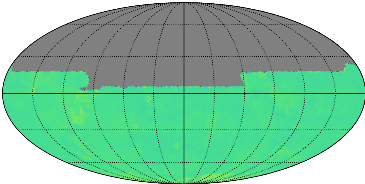
too_10_1v3.4_10yrs y: Kuiper rotTelPos
