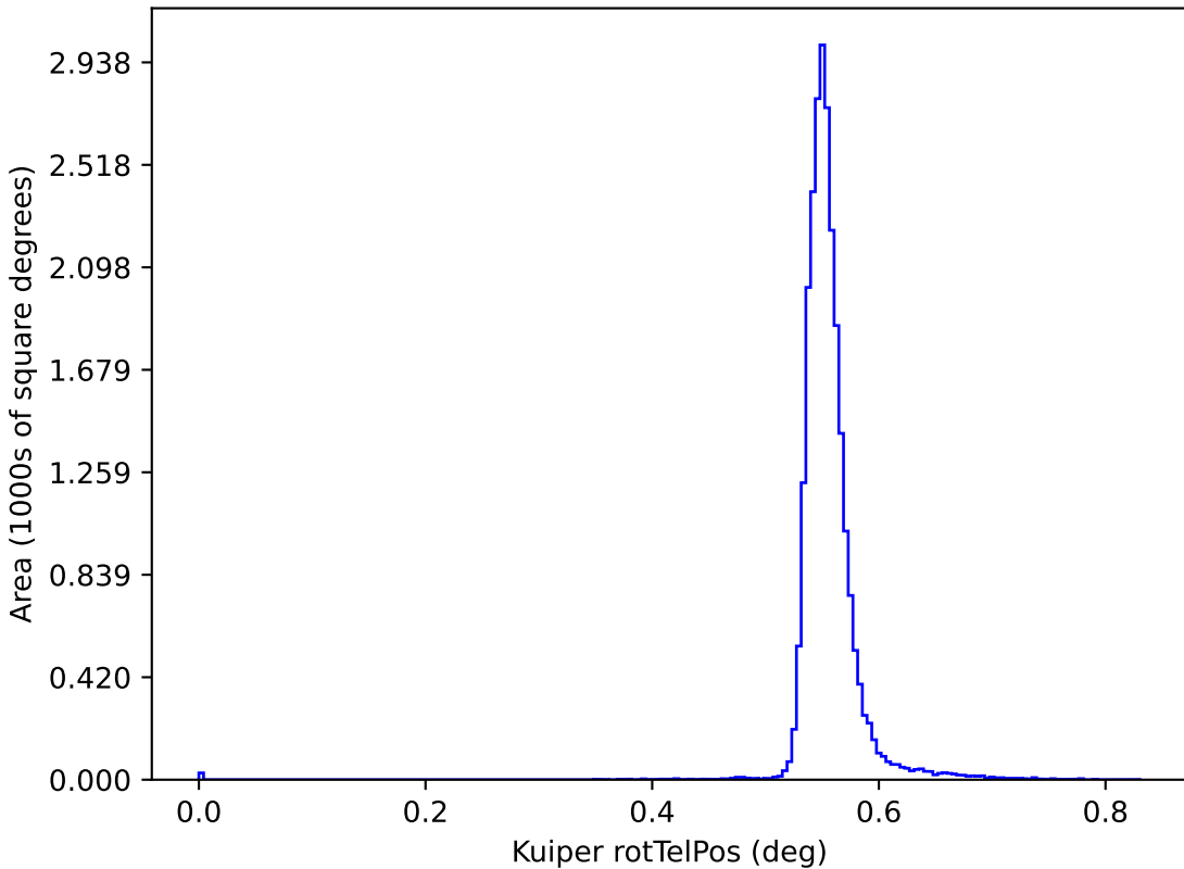
too_10_1v3.4_10yrs y: Kuiper rotTelPos
