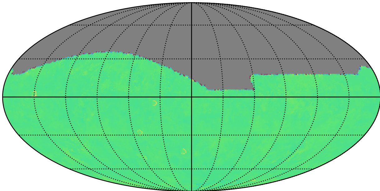
too_10_1v3.4_10yrs i: Kuiper rotTelPos
