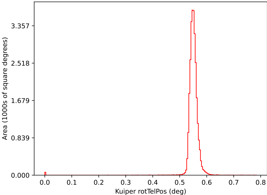
too_10_1v3.4_10yrs i: Kuiper rotTelPos
