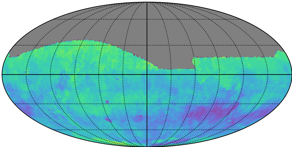
too_10_1v3.4_10yrs z: Kuiper rotSkyPos
