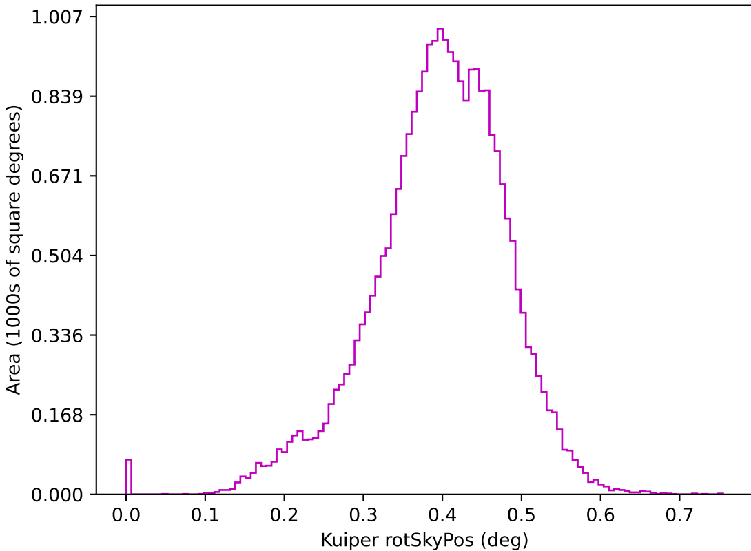
too_10_1v3.4_10yrs z: Kuiper rotSkyPos
