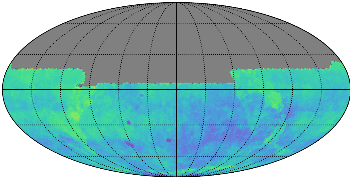
too_10_1v3.4_10yrs y: Kuiper rotSkyPos
