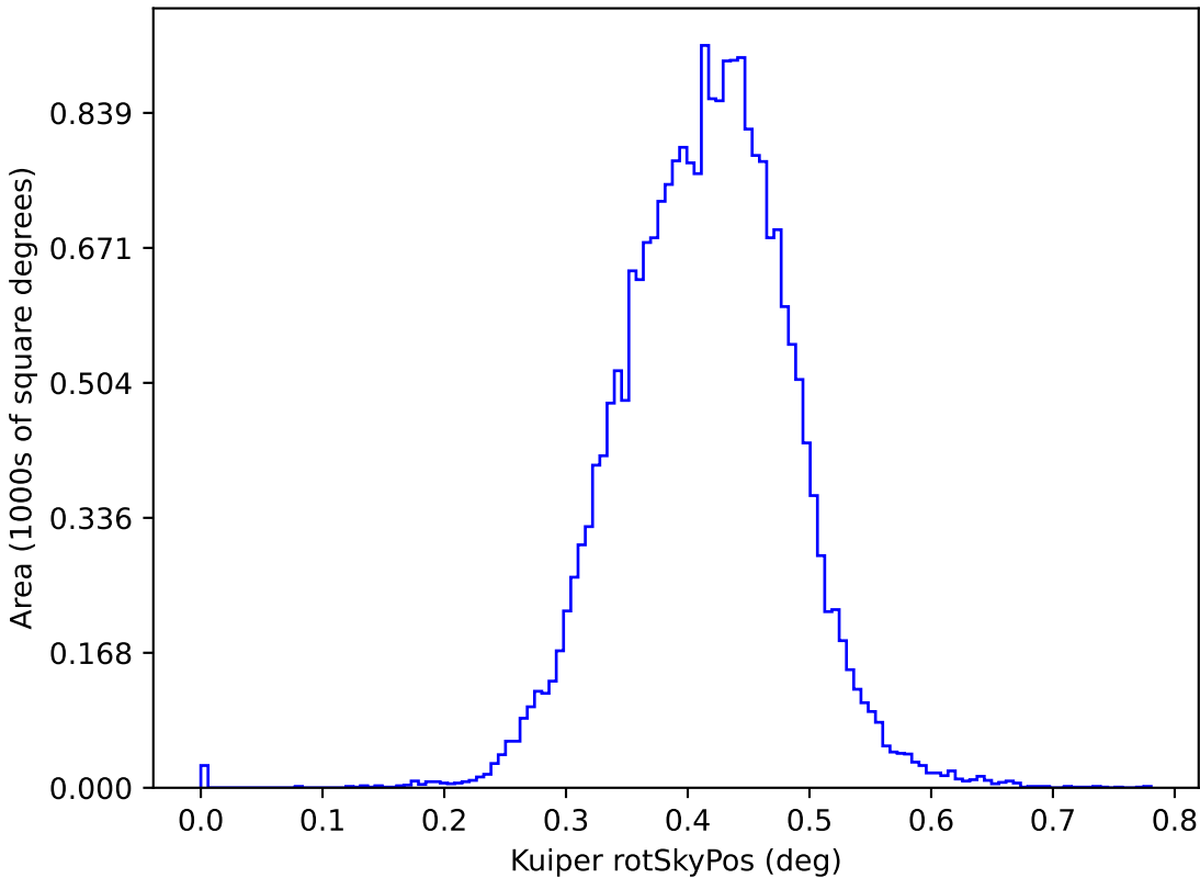
too_10_1v3.4_10yrs y: Kuiper rotSkyPos
