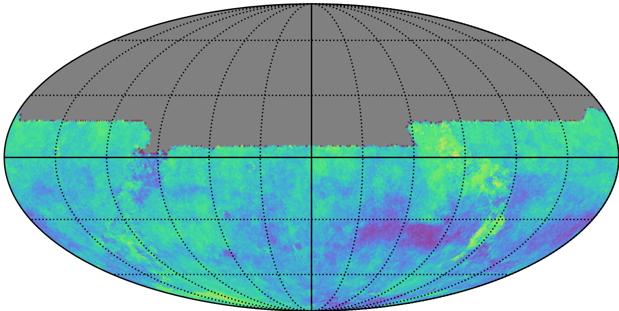
too_10_1v3.4_10yrs u: Kuiper rotSkyPos
