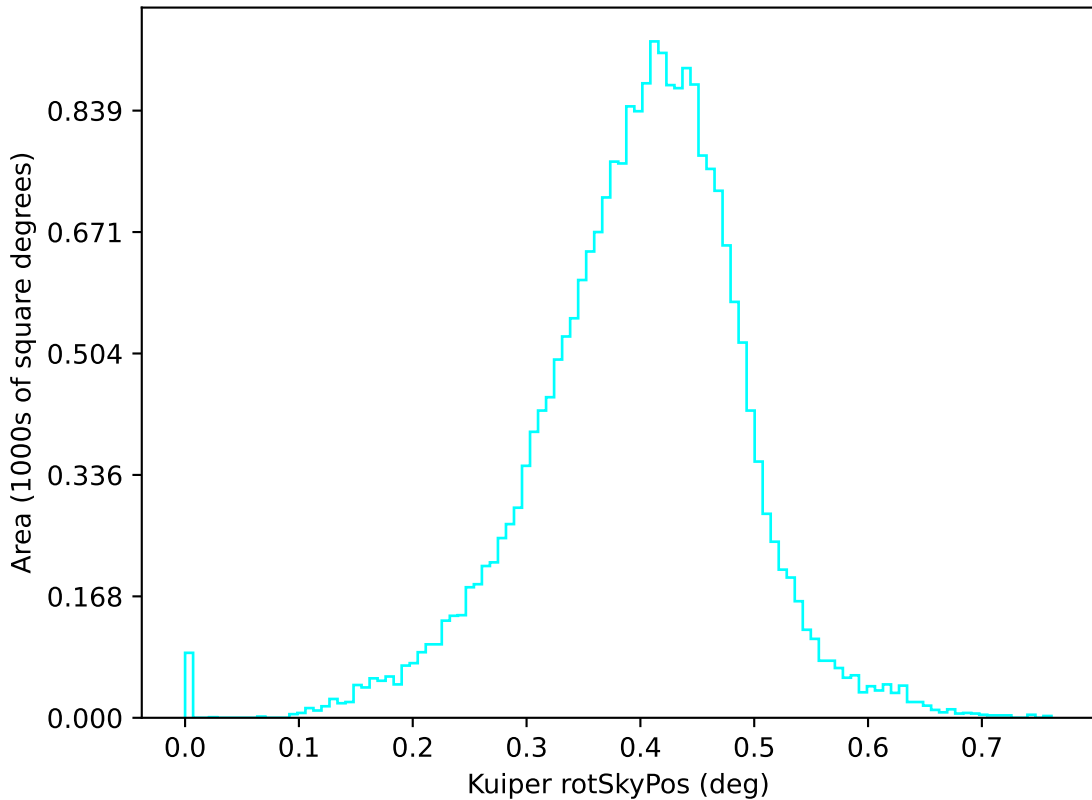
too_10_1v3.4_10yrs u: Kuiper rotSkyPos
