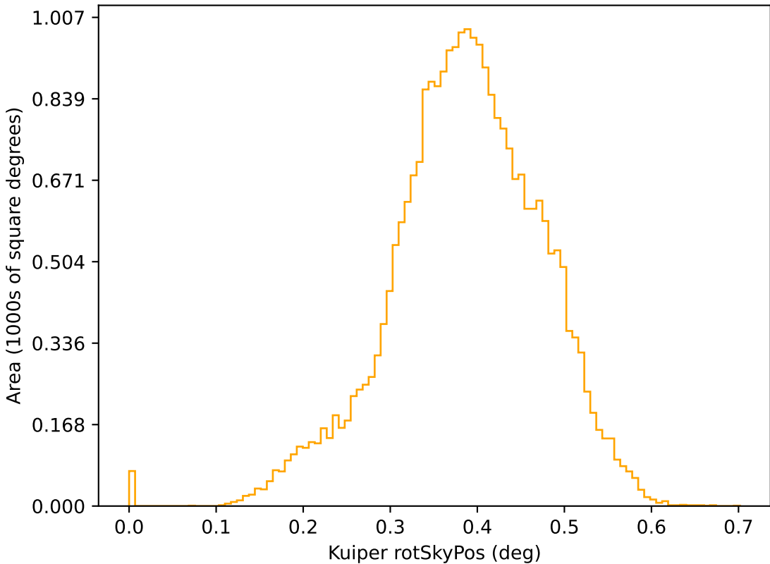
too_10_1v3.4_10yrs r: Kuiper rotSkyPos
