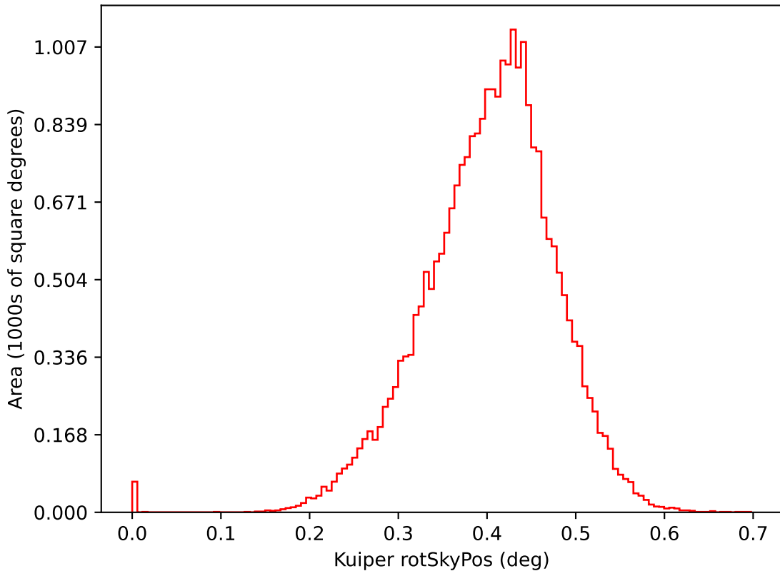
too_10_1v3.4_10yrs i: Kuiper rotSkyPos
