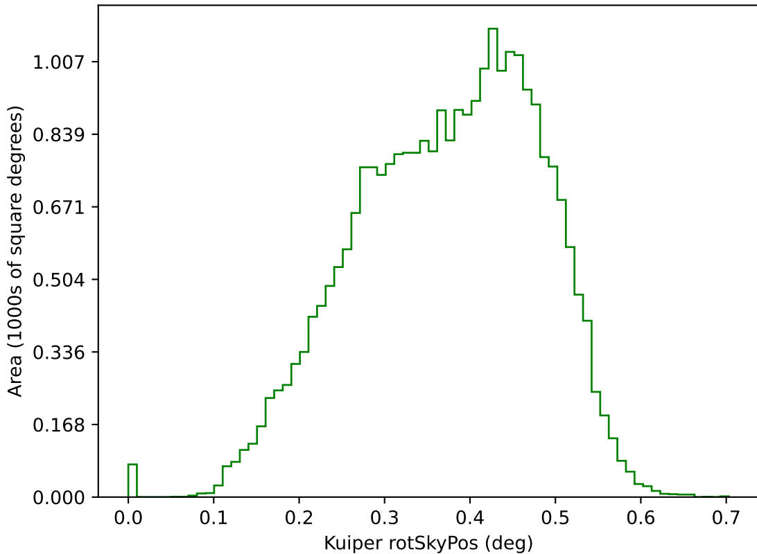
too_10_1v3.4_10yrs g: Kuiper rotSkyPos
