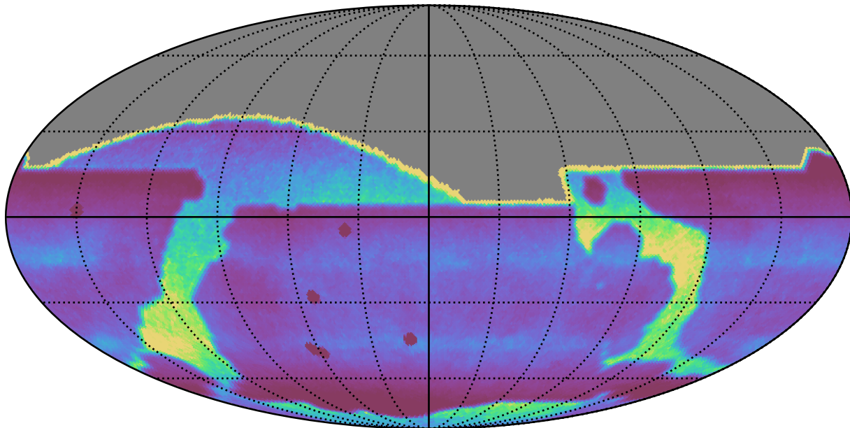
too_10_1v3.4_10yrs : DCRprecision
