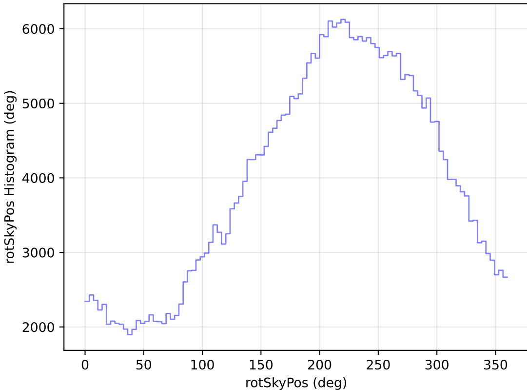
too_10_1v3.4_10yrs All sky y band: rotSkyPos Histogram
