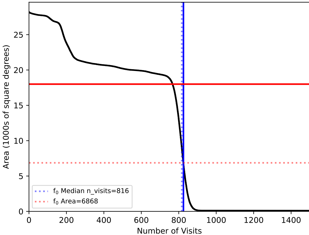
too_10_1v3.4_10yrs All sky: f0
