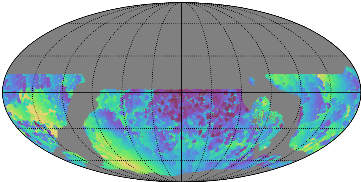
too_10_1v3.4_10yrs WFD y band: Min solarElong
