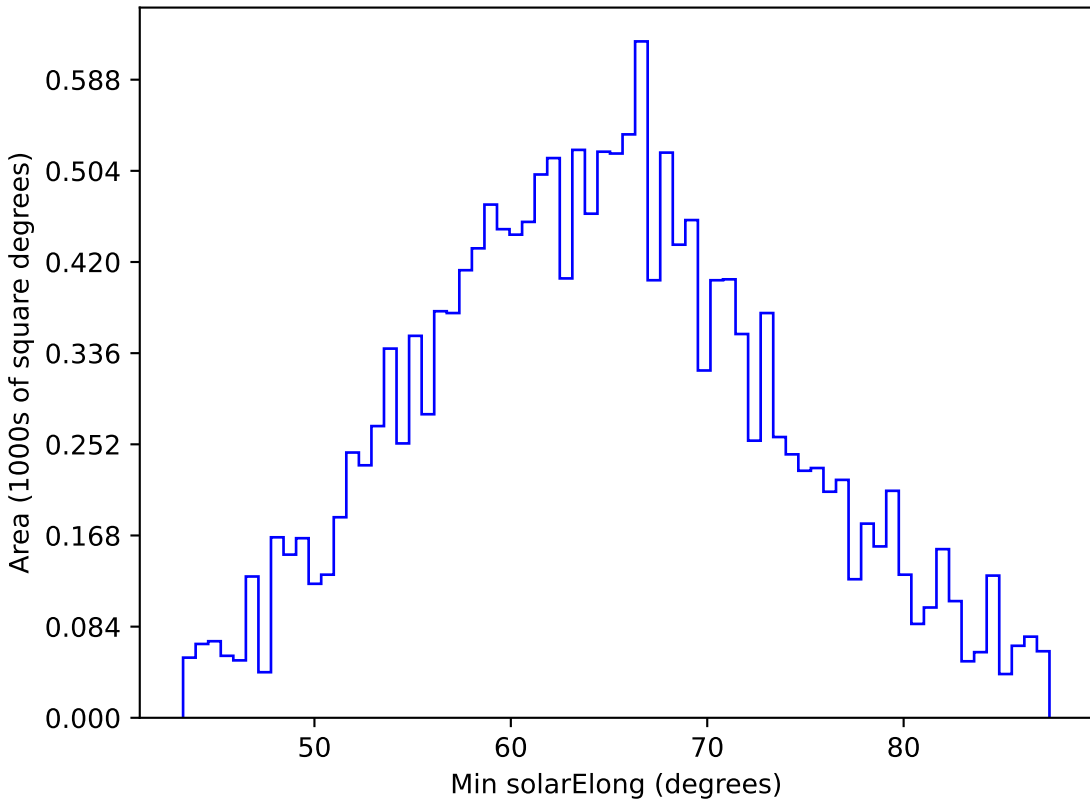
too_10_1v3.4_10yrs WFD y band: Min solarElong
