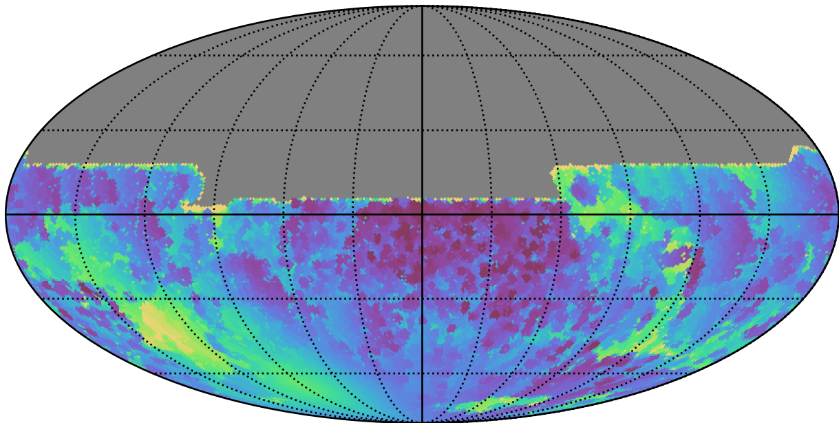
too_10_1v3.4_10yrs All sky y band: Min solarElong
