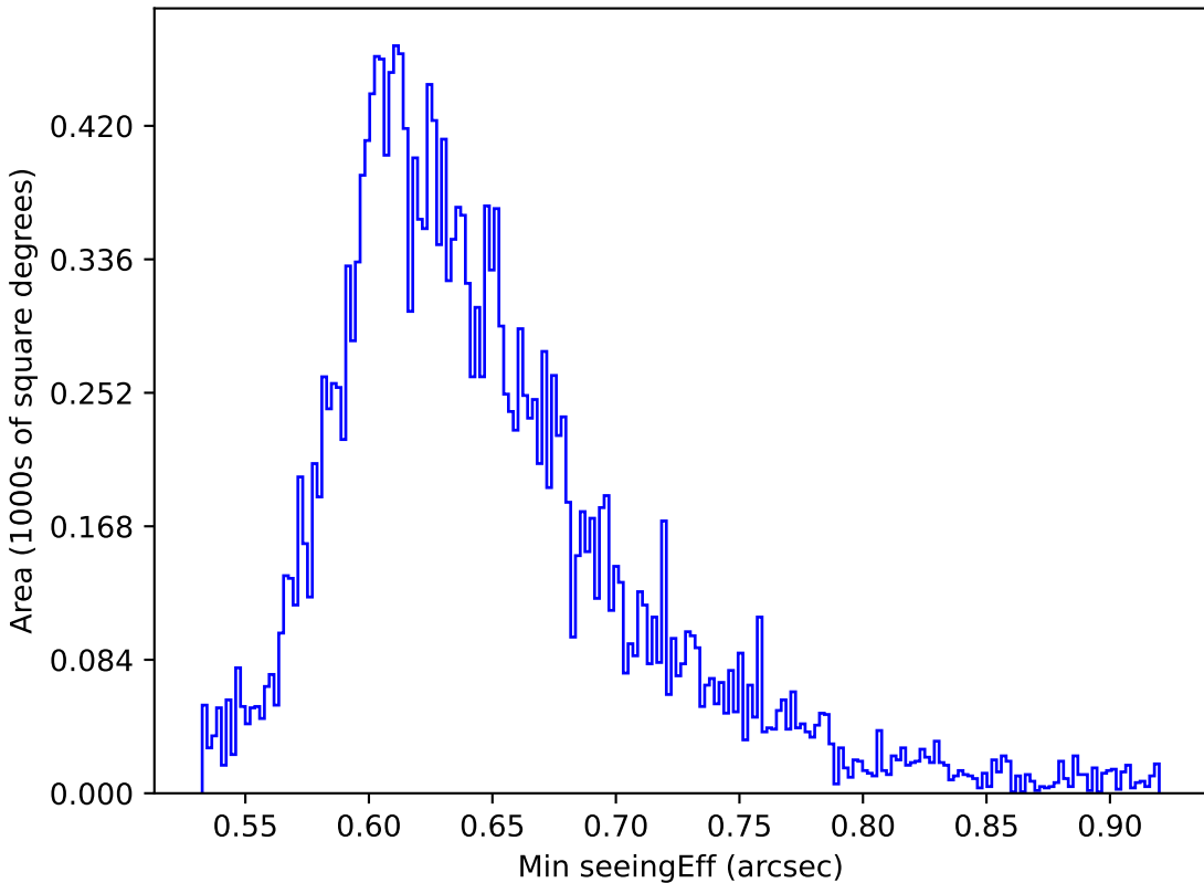
too_10_1v3.4_10yrs All sky y band: Min seeingEff
