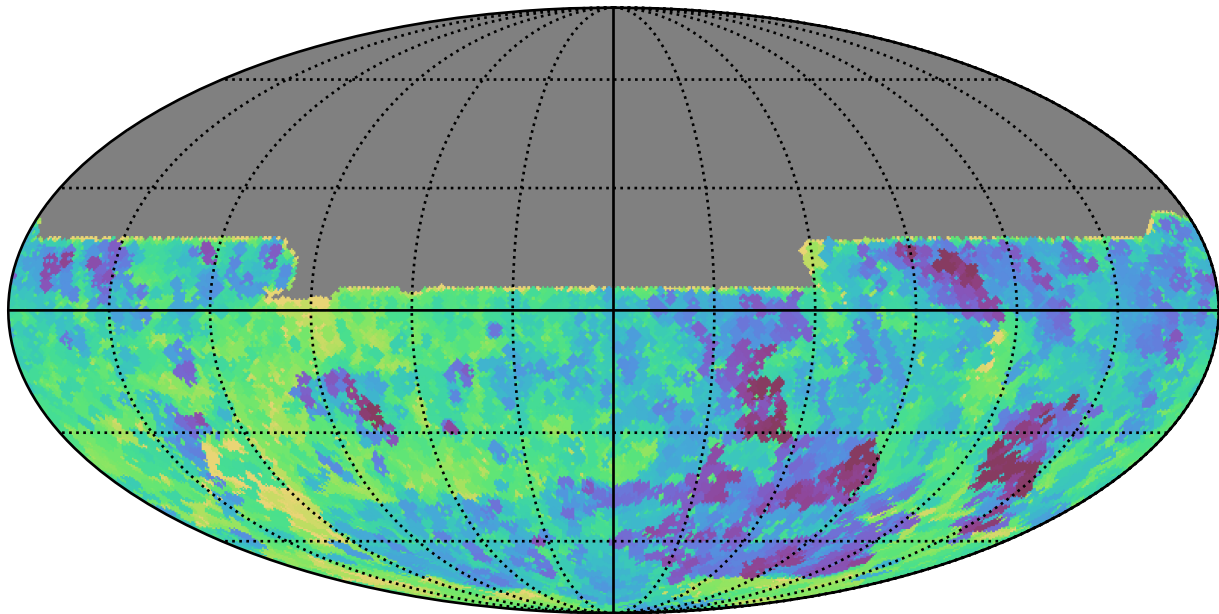
too_10_1v3.4_10yrs All sky y band: Min saturation_mag
