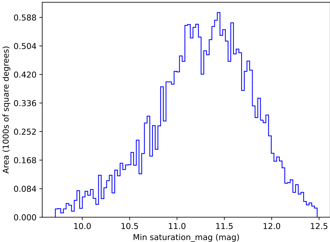
too_10_1v3.4_10yrs All sky y band: Min saturation_mag
