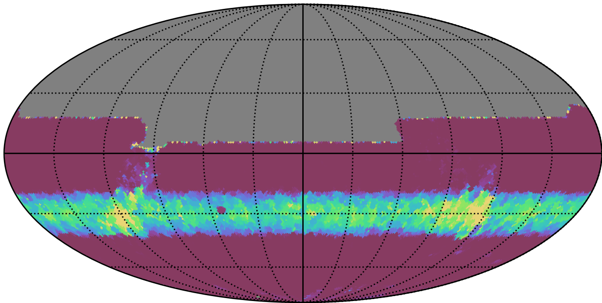
too_10_1v3.4_10yrs All sky y band: Min normairmass
