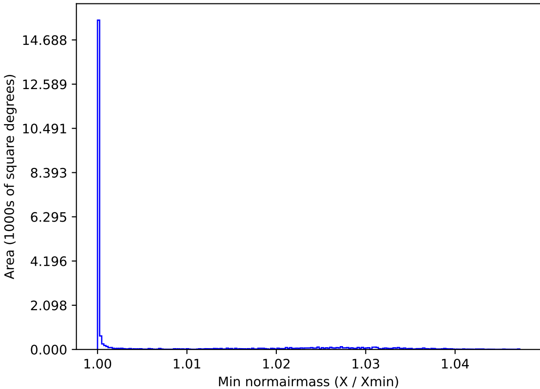
too_10_1v3.4_10yrs All sky y band: Min normairmass
