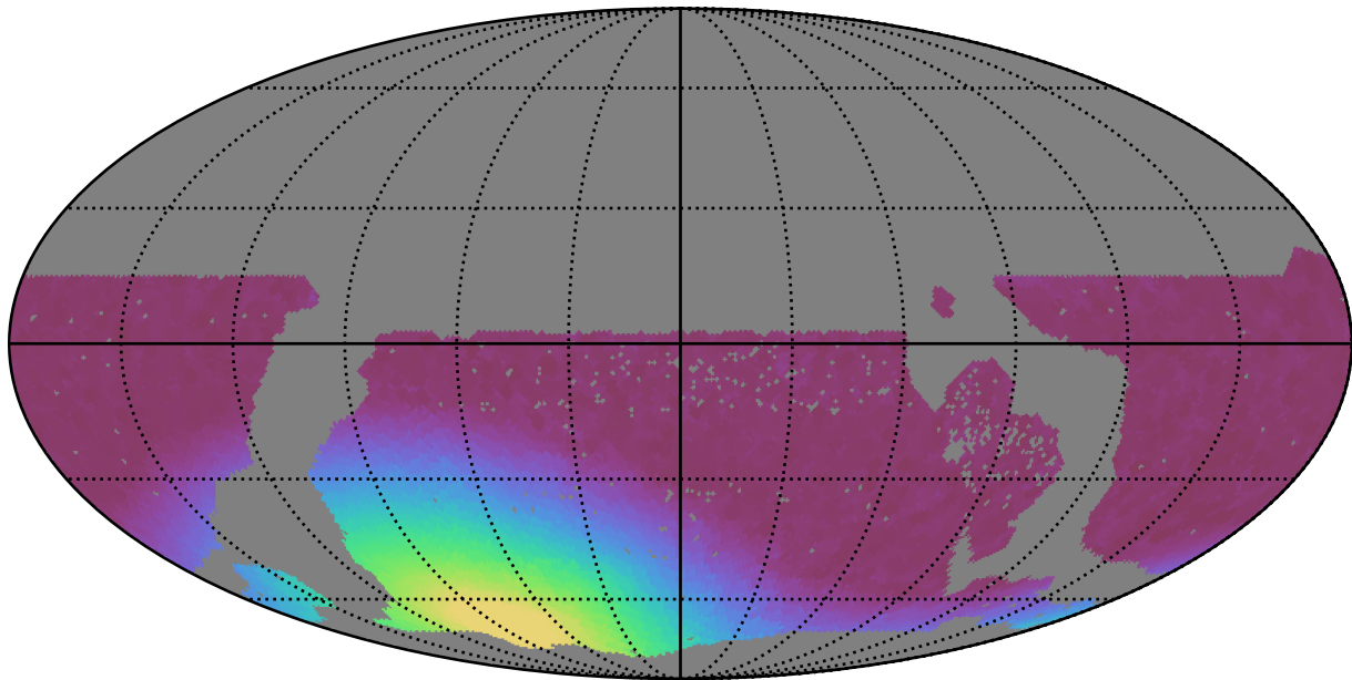
too_10_1v3.4_10yrs WFD y band: Min moonDistance
