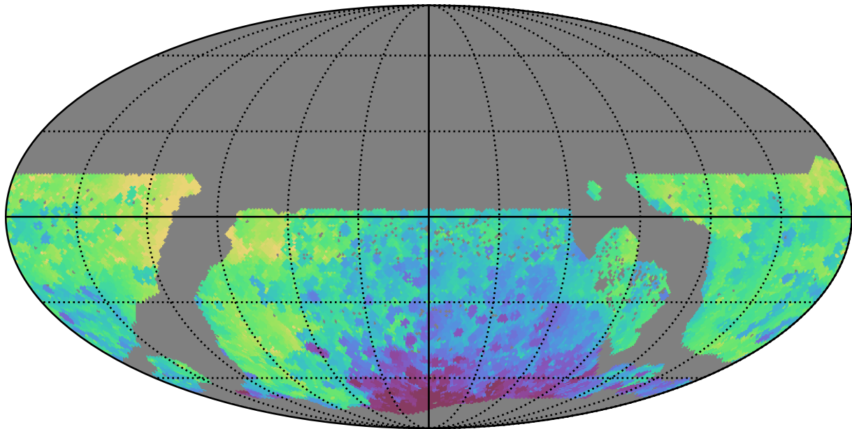
too_10_1v3.4_10yrs WFD y band: Min HA
