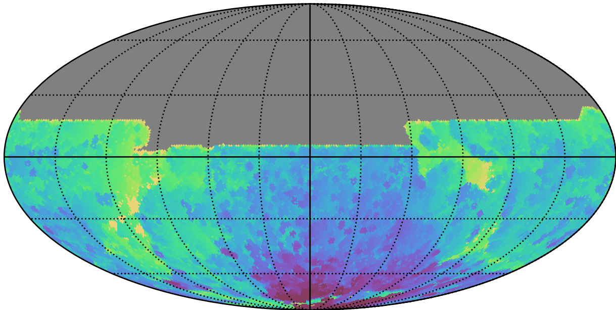
too_10_1v3.4_10yrs All sky y band: Min HA
