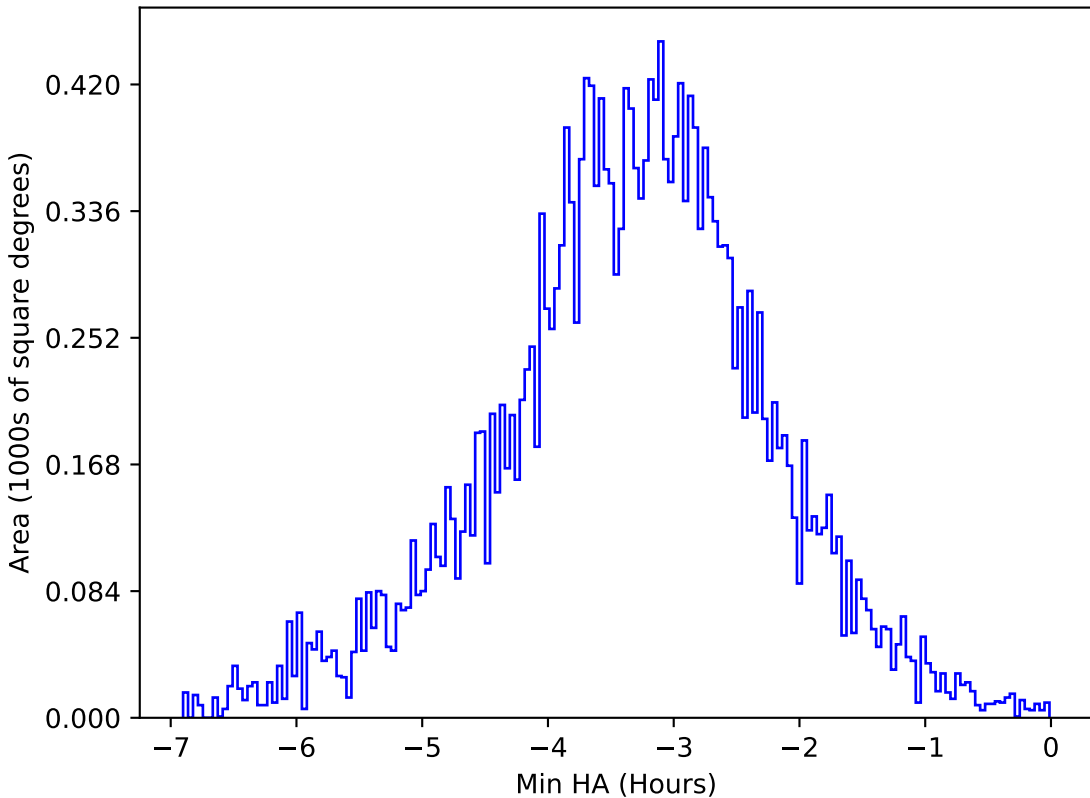
too_10_1v3.4_10yrs All sky y band: Min HA
