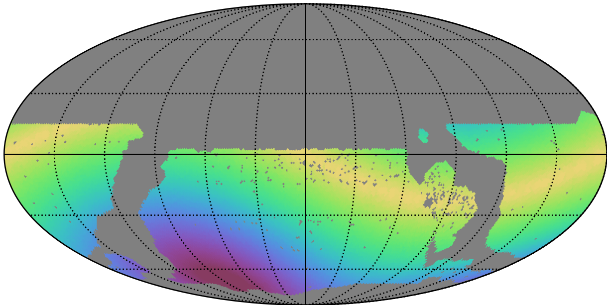
too_10_1v3.4_10yrs WFD y band: Max solarElong
