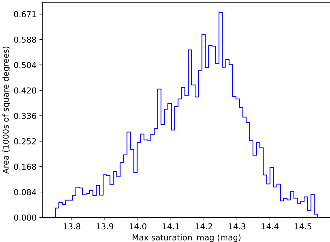
too_10_1v3.4_10yrs WFD y band: Max saturation_mag
