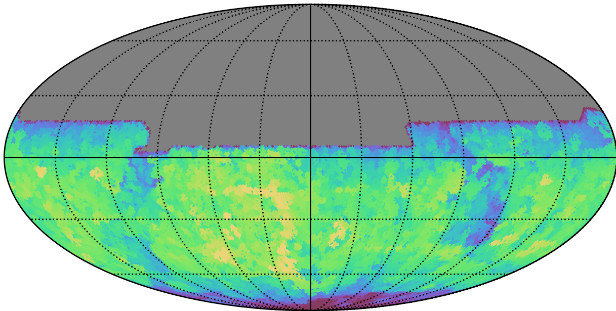
too_10_1v3.4_10yrs All sky y band: Max saturation_mag
