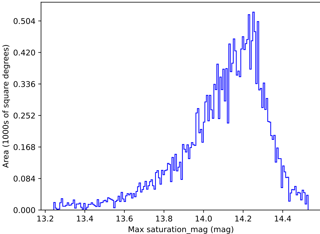
too_10_1v3.4_10yrs All sky y band: Max saturation_mag
