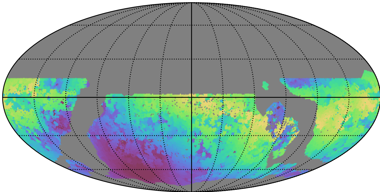
too_10_1v3.4_10yrs WFD y band: Max moonDistance
