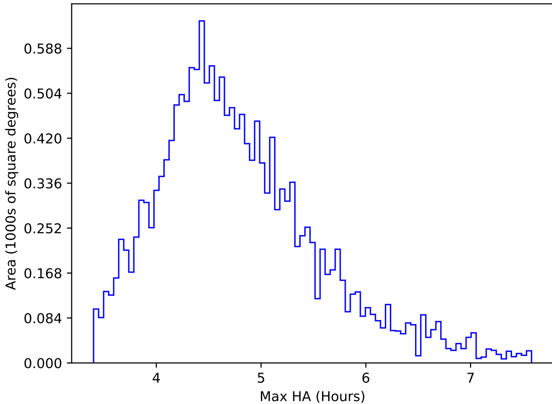
too_10_1v3.4_10yrs WFD y band: Max HA
