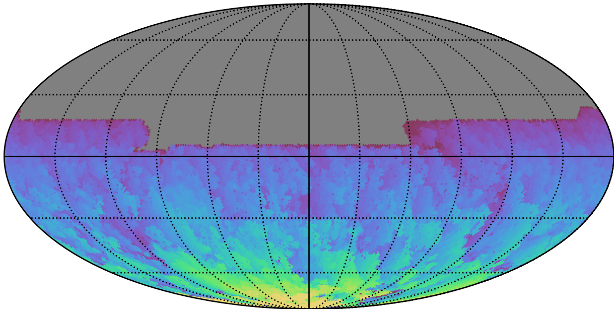
too_10_1v3.4_10yrs All sky y band: Max HA
