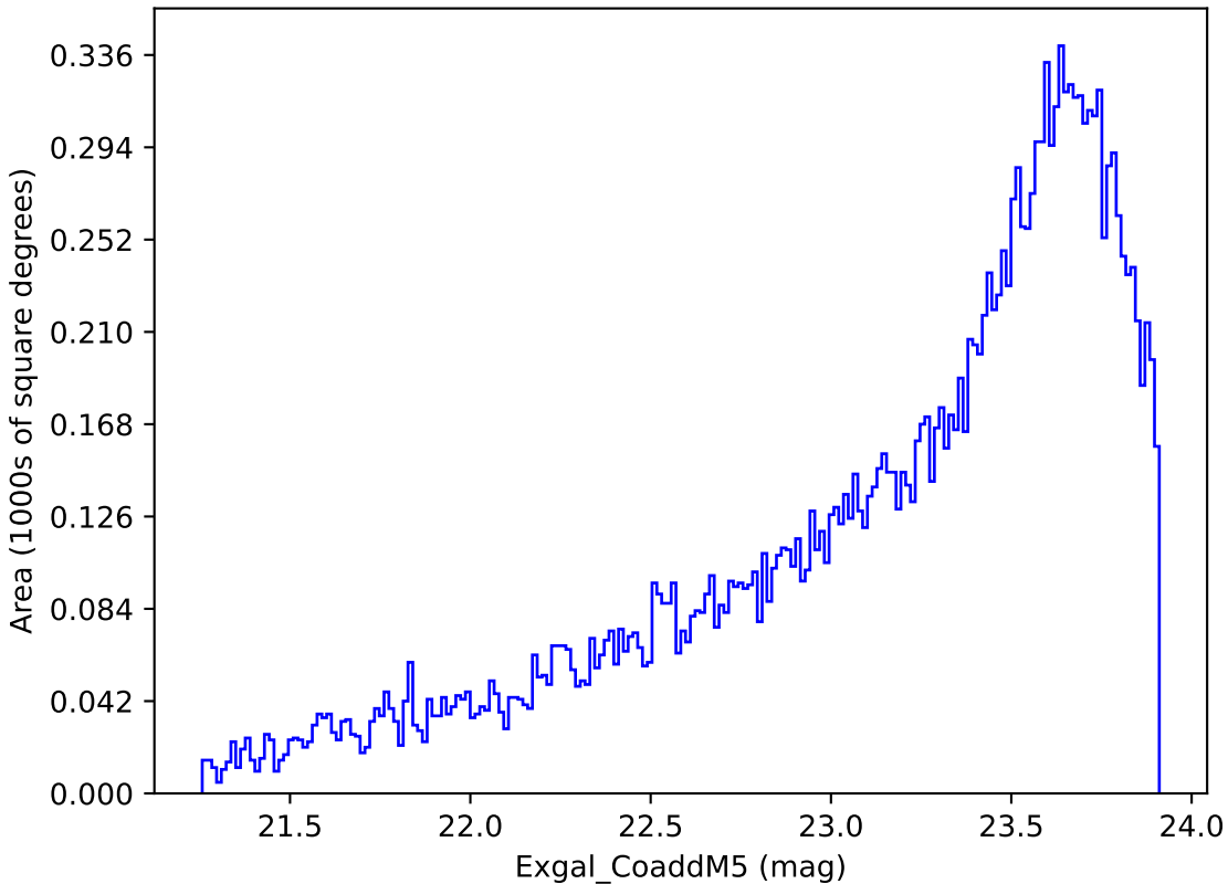
too_10_1v3.4_10yrs Yr 3-4 y band: Exgal_CoaddM5
