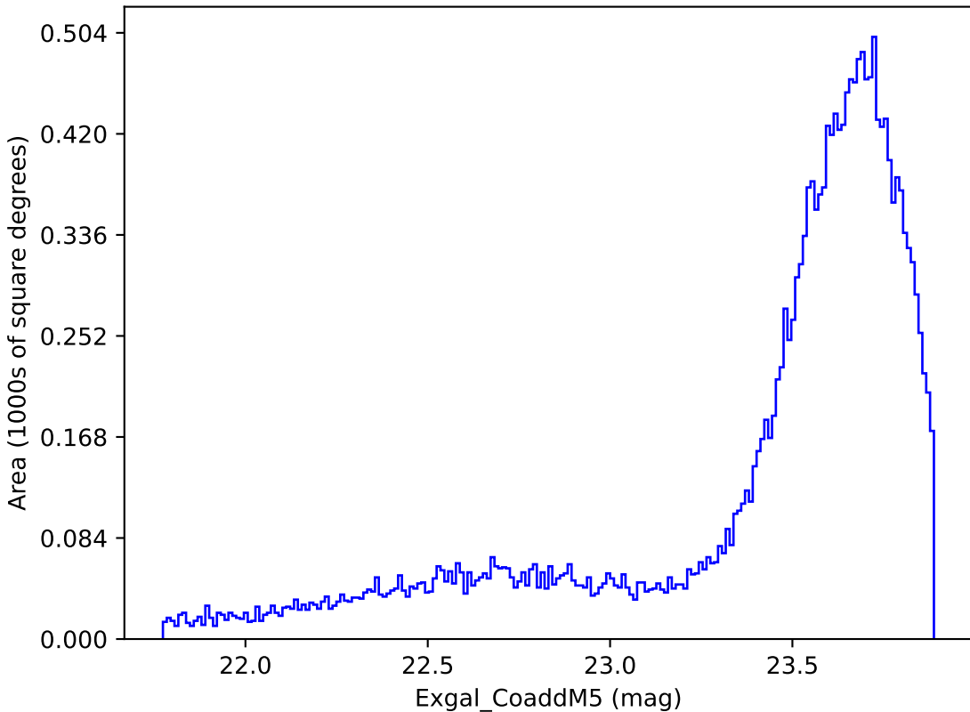
too_10_1v3.4_10yrs Yr 1 y band: Exgal_CoaddM5
