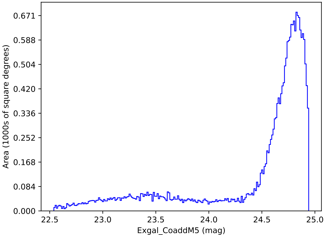
too_10_1v3.4_10yrs All sky y band: Exgal_CoaddM5
