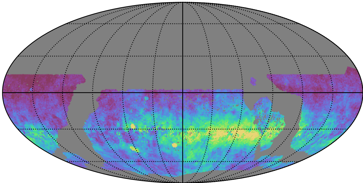
too_10_1v3.4_10yrs WFD y band: AngleRms rotSkyPos
