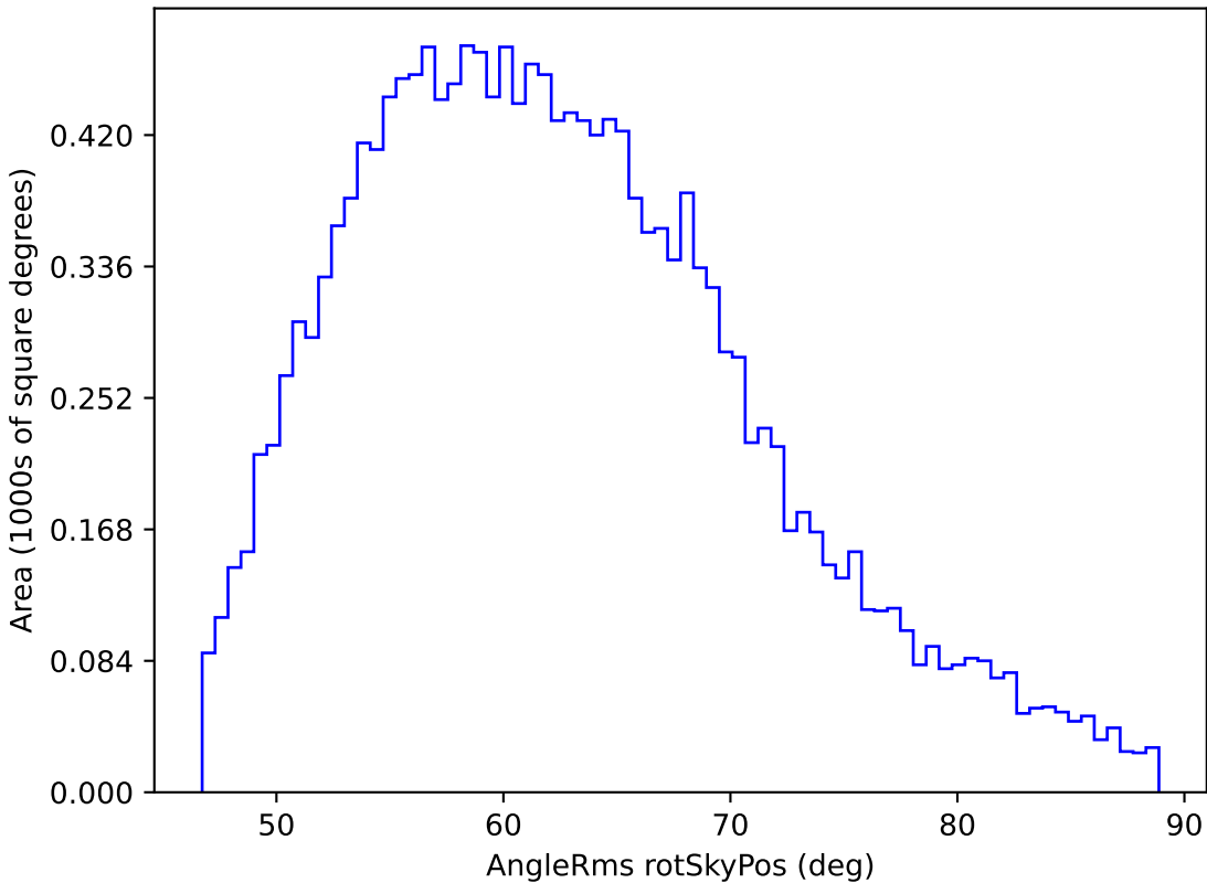
too_10_1v3.4_10yrs WFD y band: AngleRms rotSkyPos
