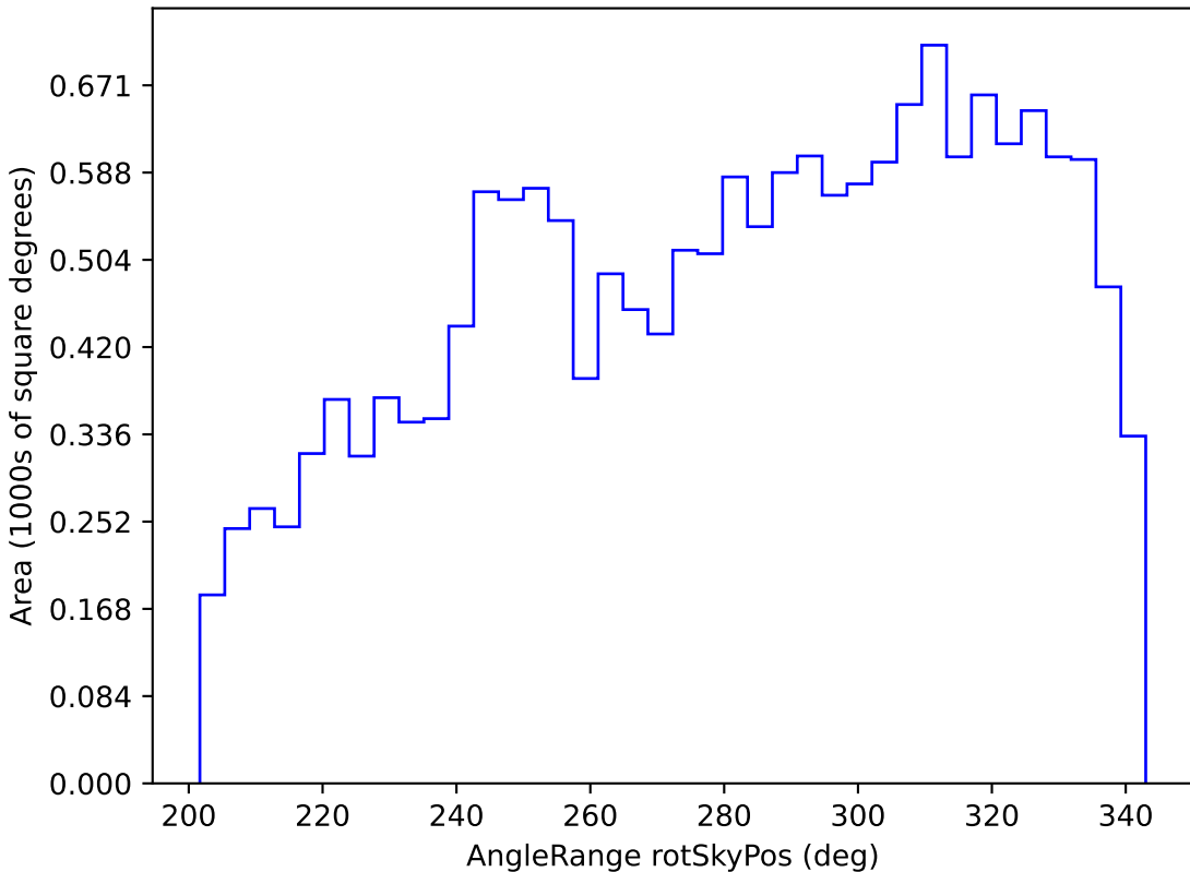
too_10_1v3.4_10yrs WFD z band: AngleRange rotSkyPos
