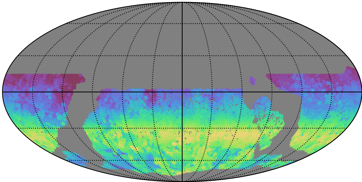
too_10_1v3.4_10yrs WFD y band: AngleRange rotSkyPos
