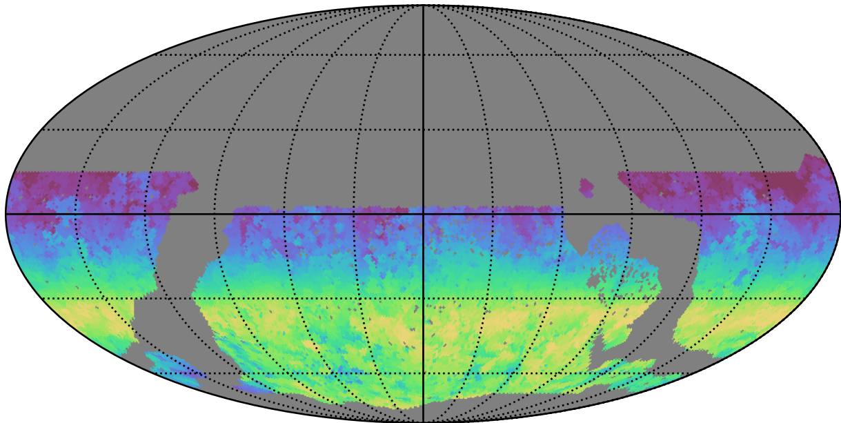
too_10_1v3.4_10yrs WFD i band: AngleRange rotSkyPos
