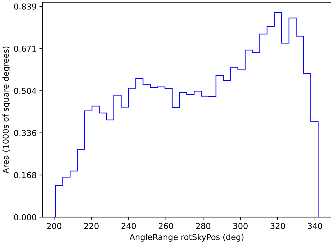
too_10_1v3.4_10yrs WFD i band: AngleRange rotSkyPos
