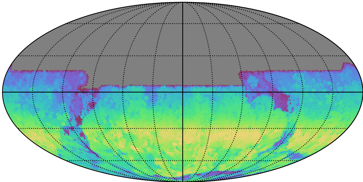
too_10_1v3.4_10yrs All sky y band: AngleRange rotSkyPos
