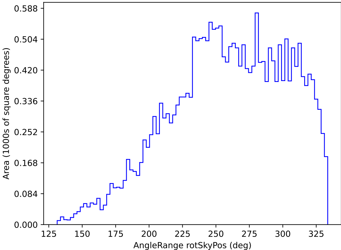
too_10_1v3.4_10yrs All sky y band: AngleRange rotSkyPos
