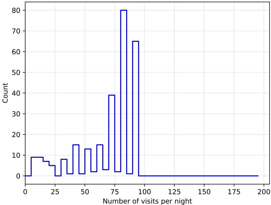
too_10_1v3.4_10yrs all bands: DD:ELAISS1 NVisitsPerNight
