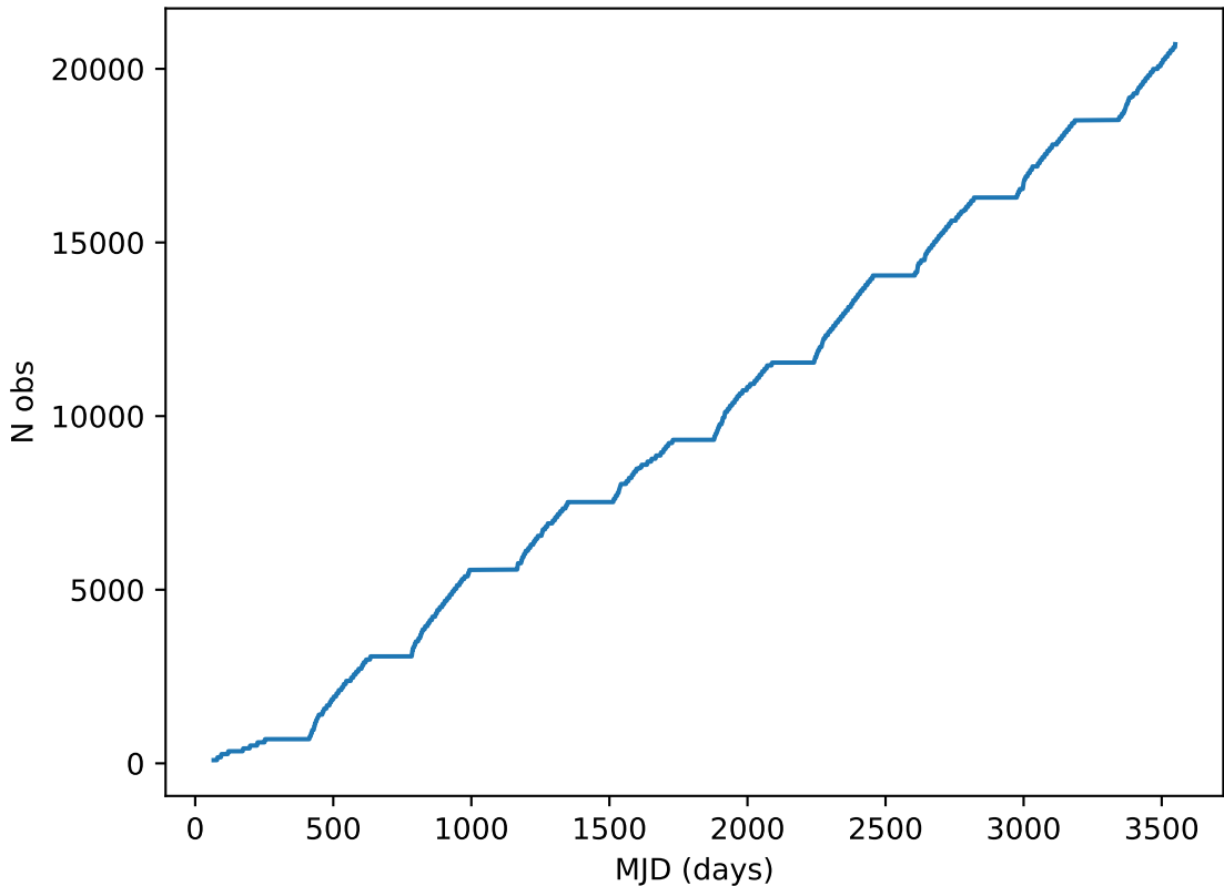
too_10_1v3.4_10yrs all bands: DD:ELAISS1 Cumulative NVisits
